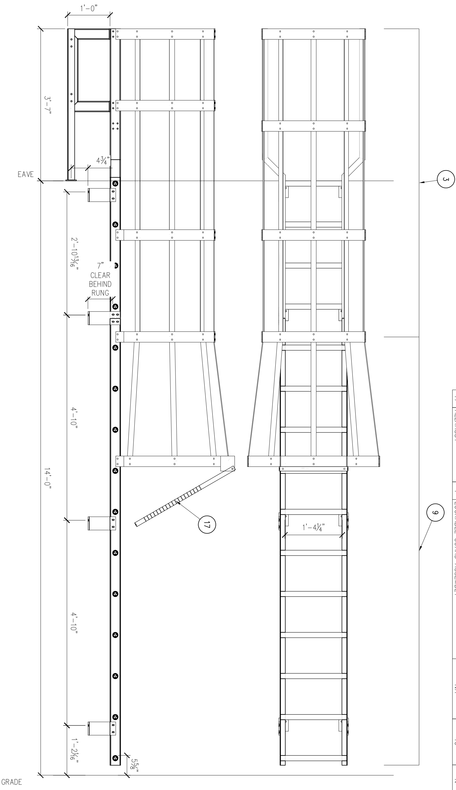
1 LADDER ASSEMBLY SCALE: 1/8" = 1'-0"
